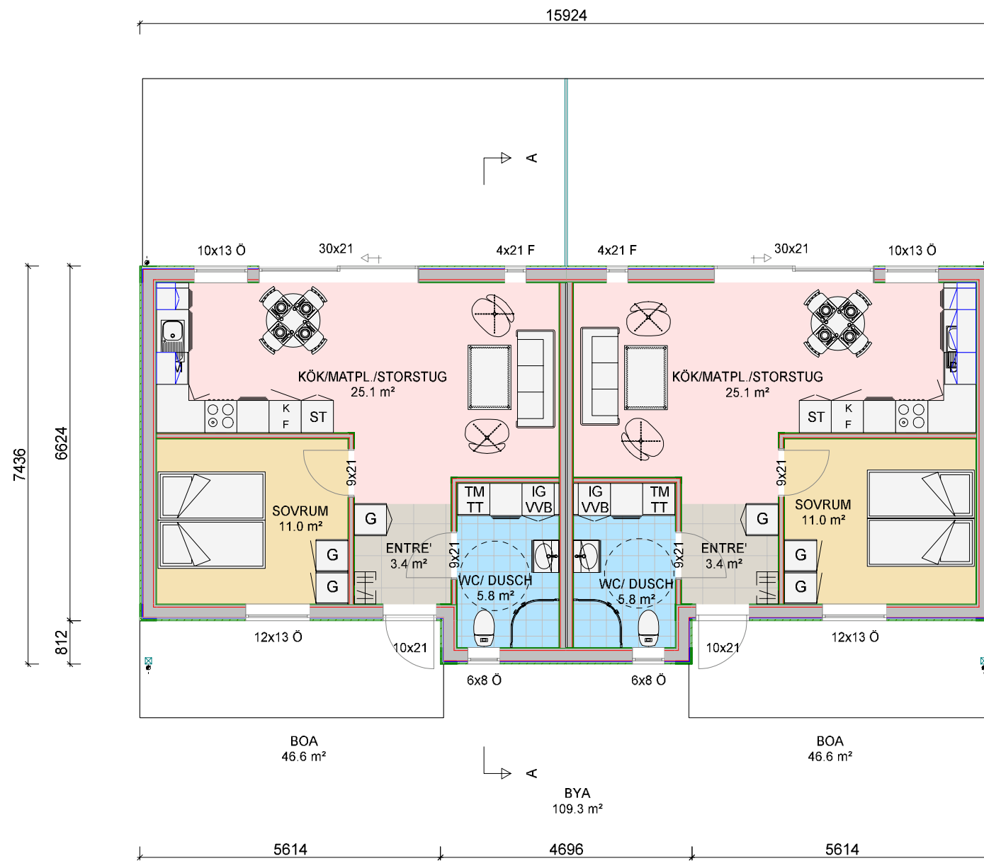
Bottenvåning
