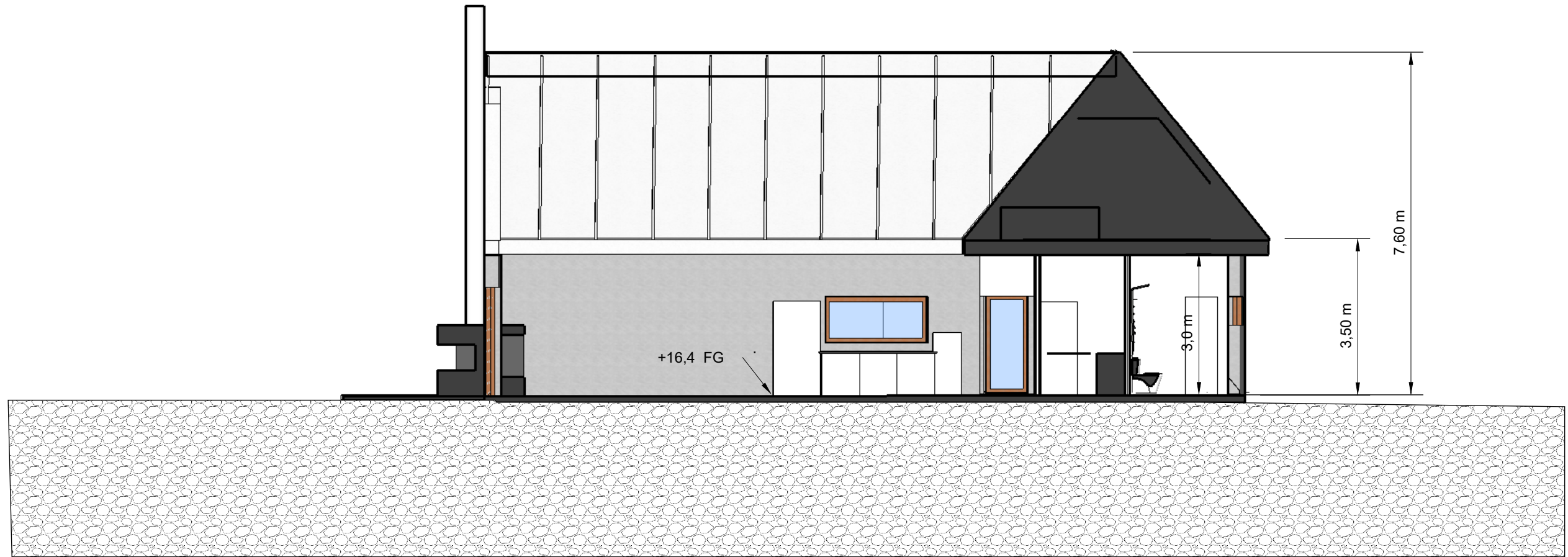
SEKTION 4-4 SKALA 1:100
