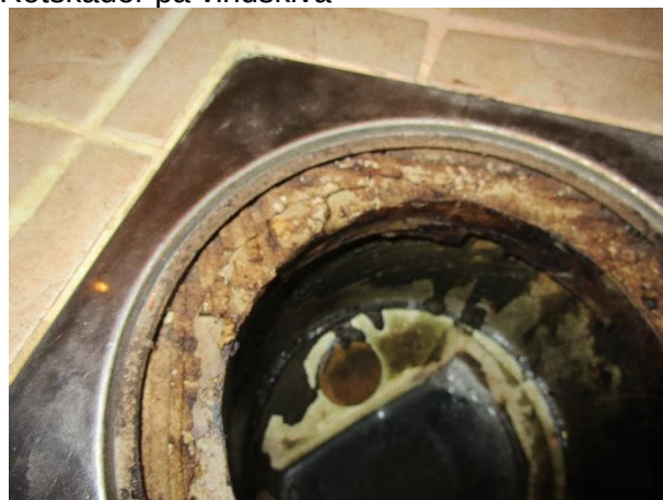
Fog och fix täcker anslutningen till klämring
